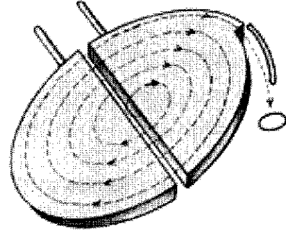
सायक्लोट्रॉन
